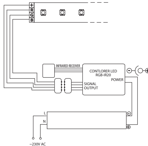
Przykładowy schemat układu zasilania oraz sterowania barwą liniowych modułów LED RGB LED RGB line modules feed system and colour controlling wiring diagram
